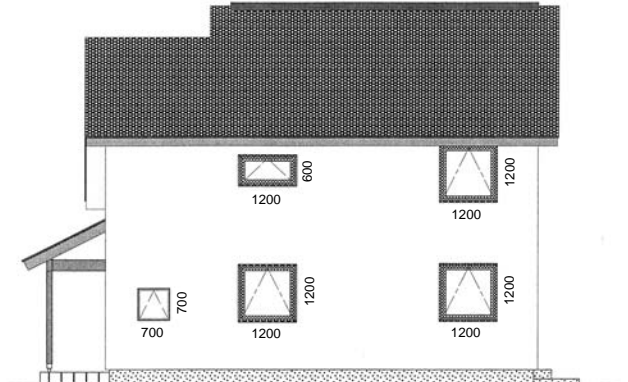
西側立面図
