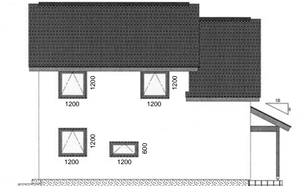
東側立面図
